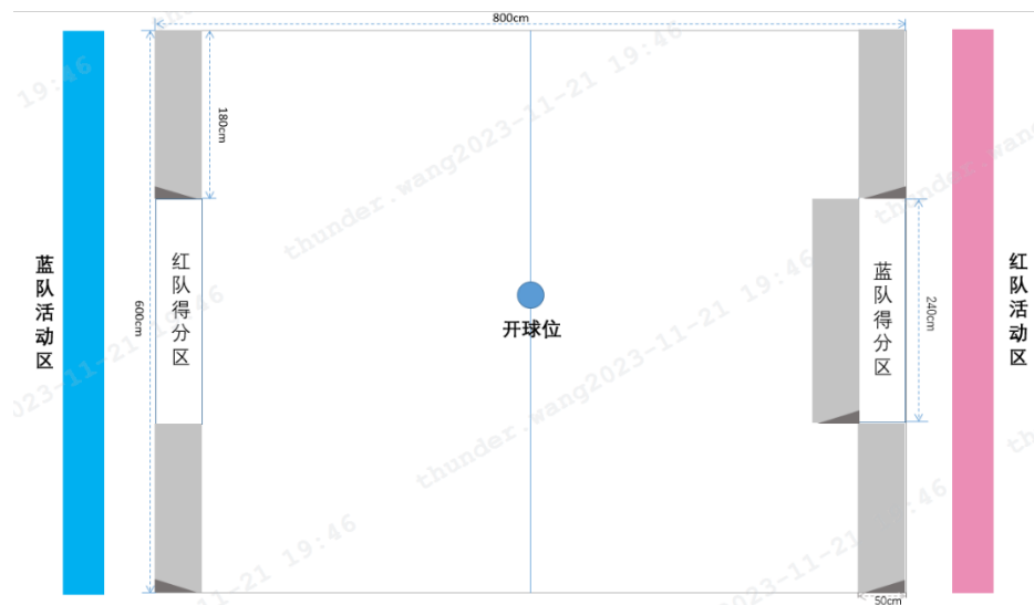
6. 飞行区场地尺寸图（长、宽、高：6m×8m×3m）：
