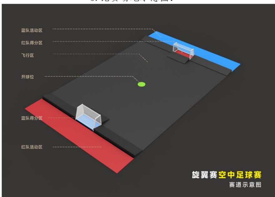
6. 飞行区场地尺寸图（长、宽、高：6m×8m×3m）：
